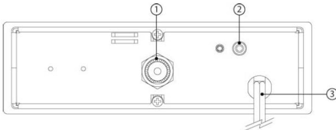
Рис. 2 Задняя панель MJ-100
