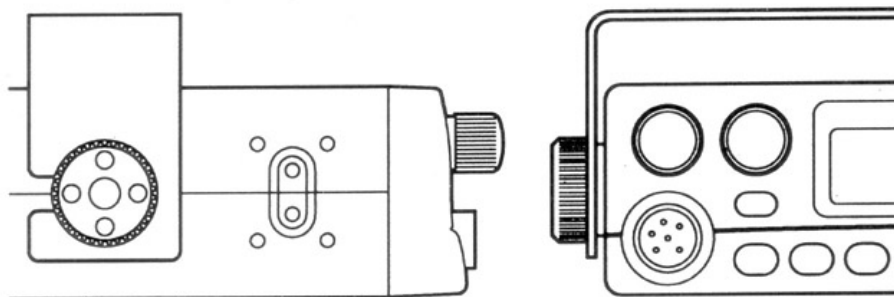
Рис. 4. Крепление радиостанции фиксаторами.
