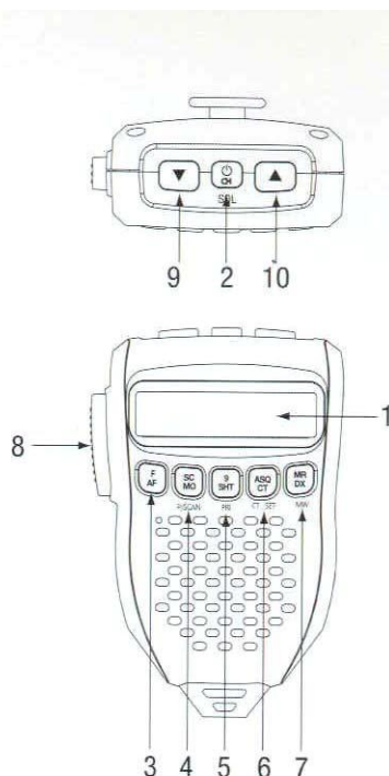
Рис. 3. Тангента радиостанции MegaJet MJ-555
